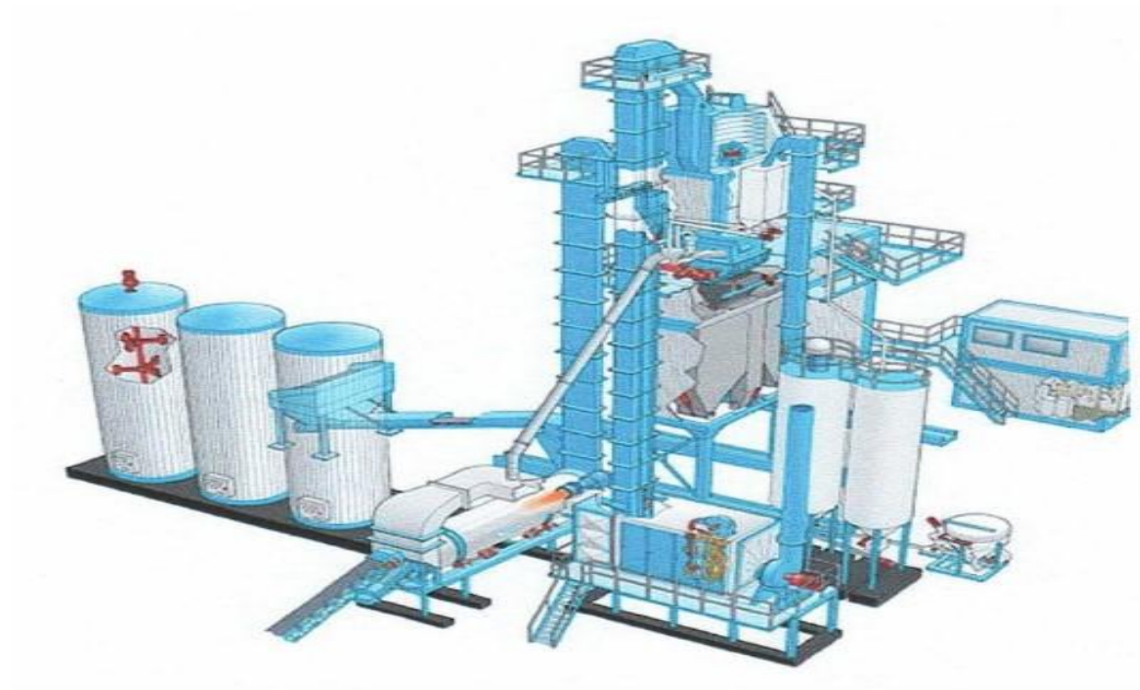
Schemat instalacji do produkcji mas bitumicznych
